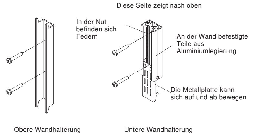
Obere Wandhalterung
