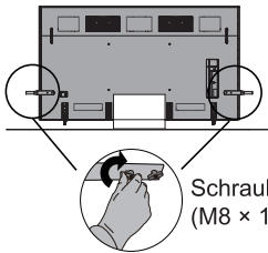
Abbildung 1 Zum Befestigen im Uhrzeigersinn drehen
